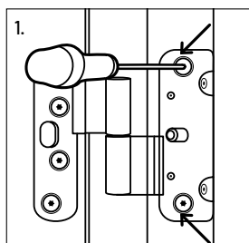
Udadgående pladedør
